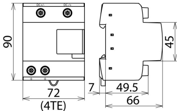
Rysunek wymiarowy DCB YPV 1200
