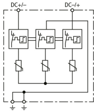
Schemat połączeń DCB YPV 1500
