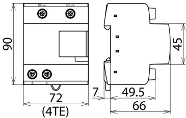
Rysunek wymiarowy DCB YPV 1500
