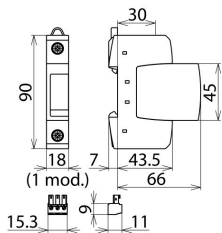
Rysunek wymiarowy DG S 150 FM
