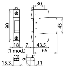
Rysunek wymiarowy DG S 385 FM
