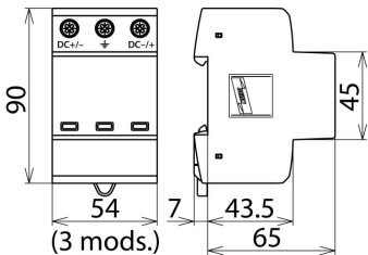
Rysunek wymiarowy DG YPV SCI 600
