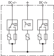
Schemat połączeń DG YPV SCI 1000
