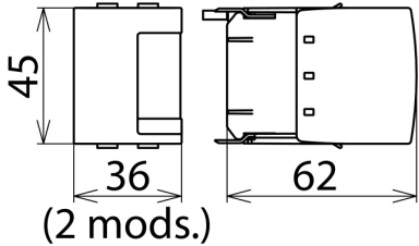
Rysunek wymiarowy DB M MOD 150
