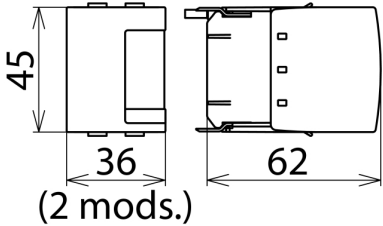
Rysunek wymiarowy DB M MOD 255
