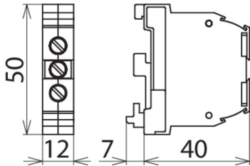
Rysunek wymiarowy SLK 16
