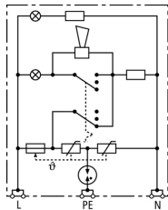
Schemat połączeń DSA 230 LA
