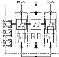
Schemat połączeń DG ME YPV SCI1500 FM
