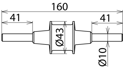
Rysunek wymiarowy KFSU
