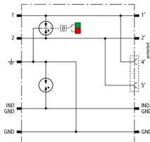
Schemat połączeń DBX TC B 180
