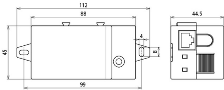
Rysunek wymiarowy DBX TC B 180
