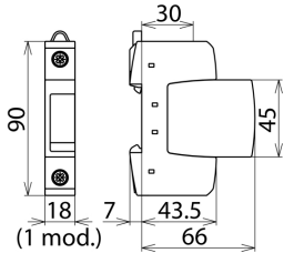
Rysunek wymiarowy DK 25
