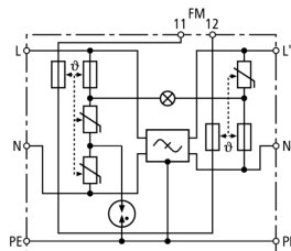
Schemat połączeń SPS PRO
