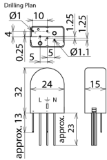
Rysunek wymiarowy VC 280 2
