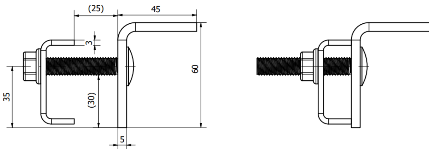
Rys.1 Wymiary uchwytu K-24-U
