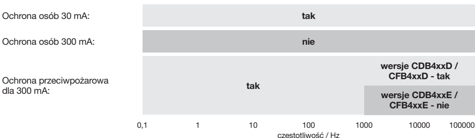
Schemat ochrony przeciwporażeniowej oraz przeciwpożarowej dla urządzeń RCD typu B w zależności od częstotliwości.
