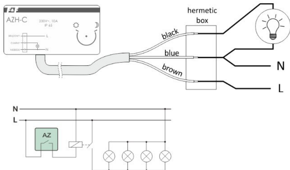
Układ sterowania stycznikiem załączającym odbiorniki o łącznym poborze prądu przewyższającym dopuszczalne obciążenie styku automatu zmierzchowego
