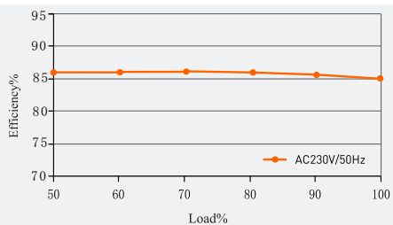
wydajność vs obciążenie / efficiency vs load
