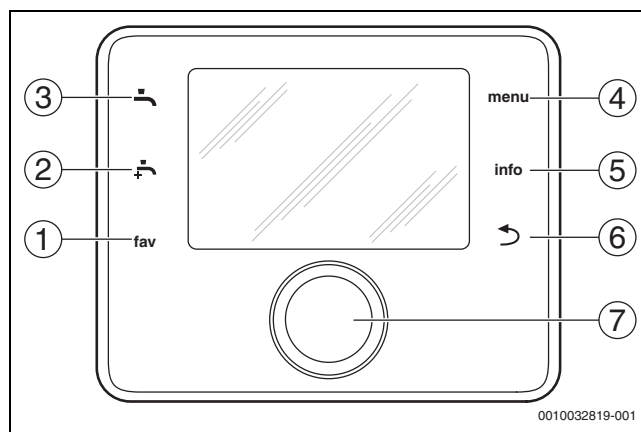
Rys. 3 Elementy obsługowe
