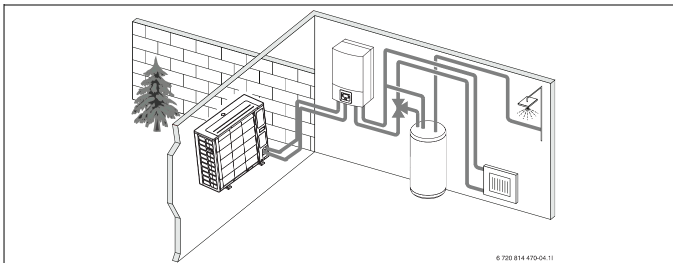
Rys. 2 Pompa ciepła jednostki zewnętrznej, jednostka wewnętrzna AWES z dogrzewaczem elektrycznym, zewnętrzny podgrzewacz pojemnościowy c.w.u.
