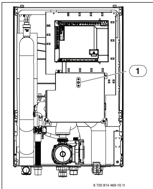
Rys. 6 Jednostka wewnętrzna AWES
