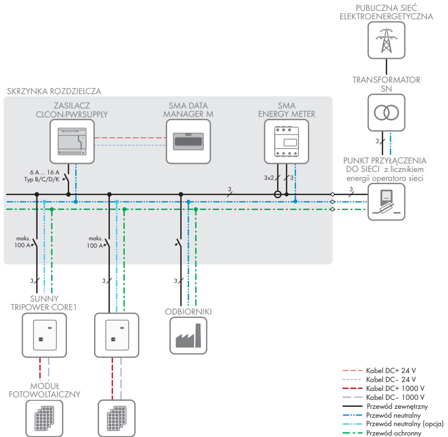
Ilustracja 4: Schemat ideowy (przykład)
