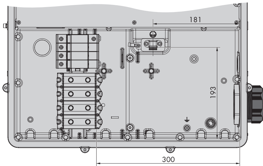
Ilustracja 11: Widok wewnętrzny podzespołu AC-Connection Unit z wymiarami dotyczącymi podłączenia przewodów (wymiary w mm)
