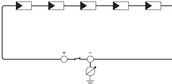
Ilustracja 19: Schemat pomiaru
