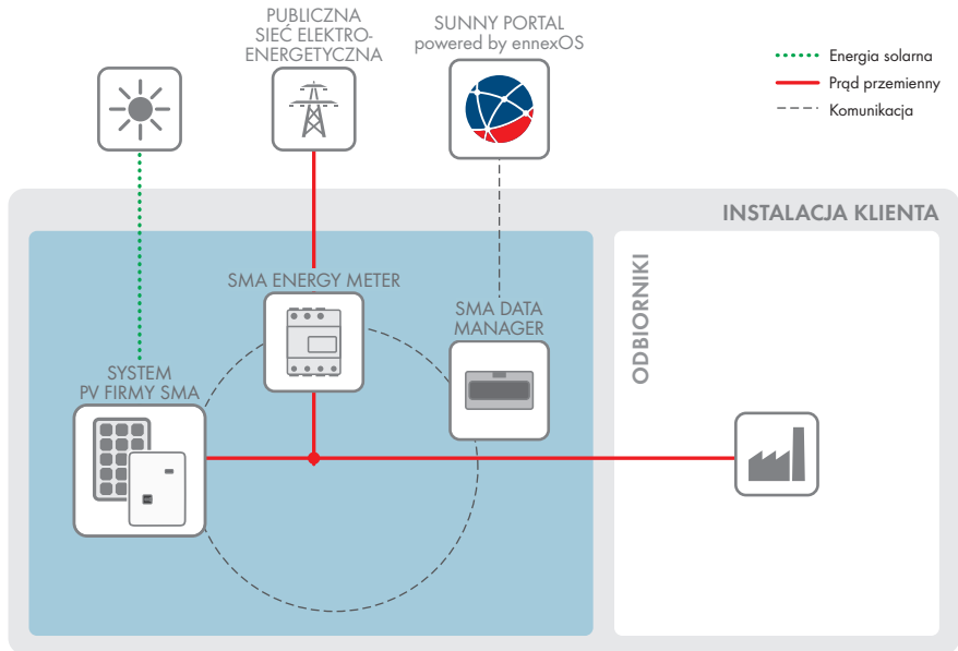
Ilustracja 3: Budowa systemu
