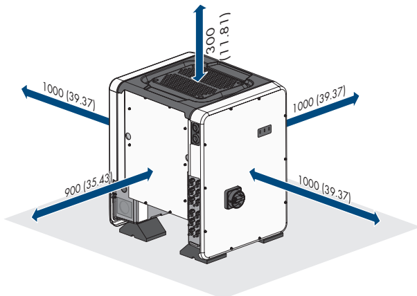
Ilustracja 9: Zalecane odstępy (wymiar w mm)
