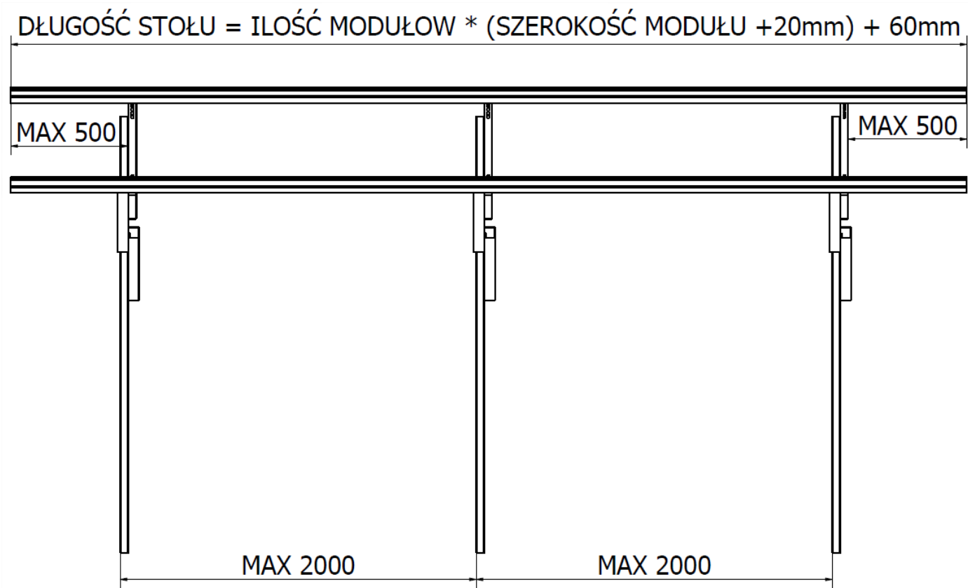
RYS.2. Długość stołu
