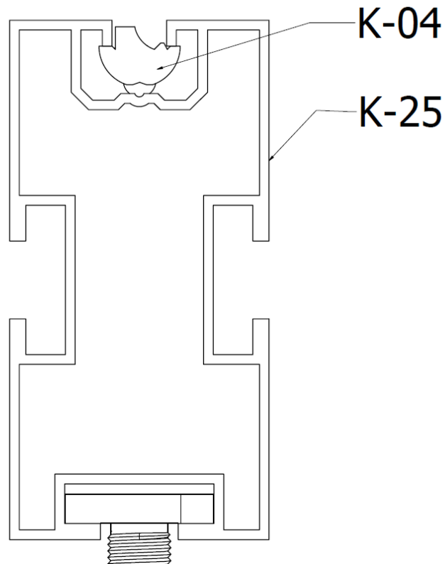
RYS.15. Montaż wpustu K-04 do profili K-25
