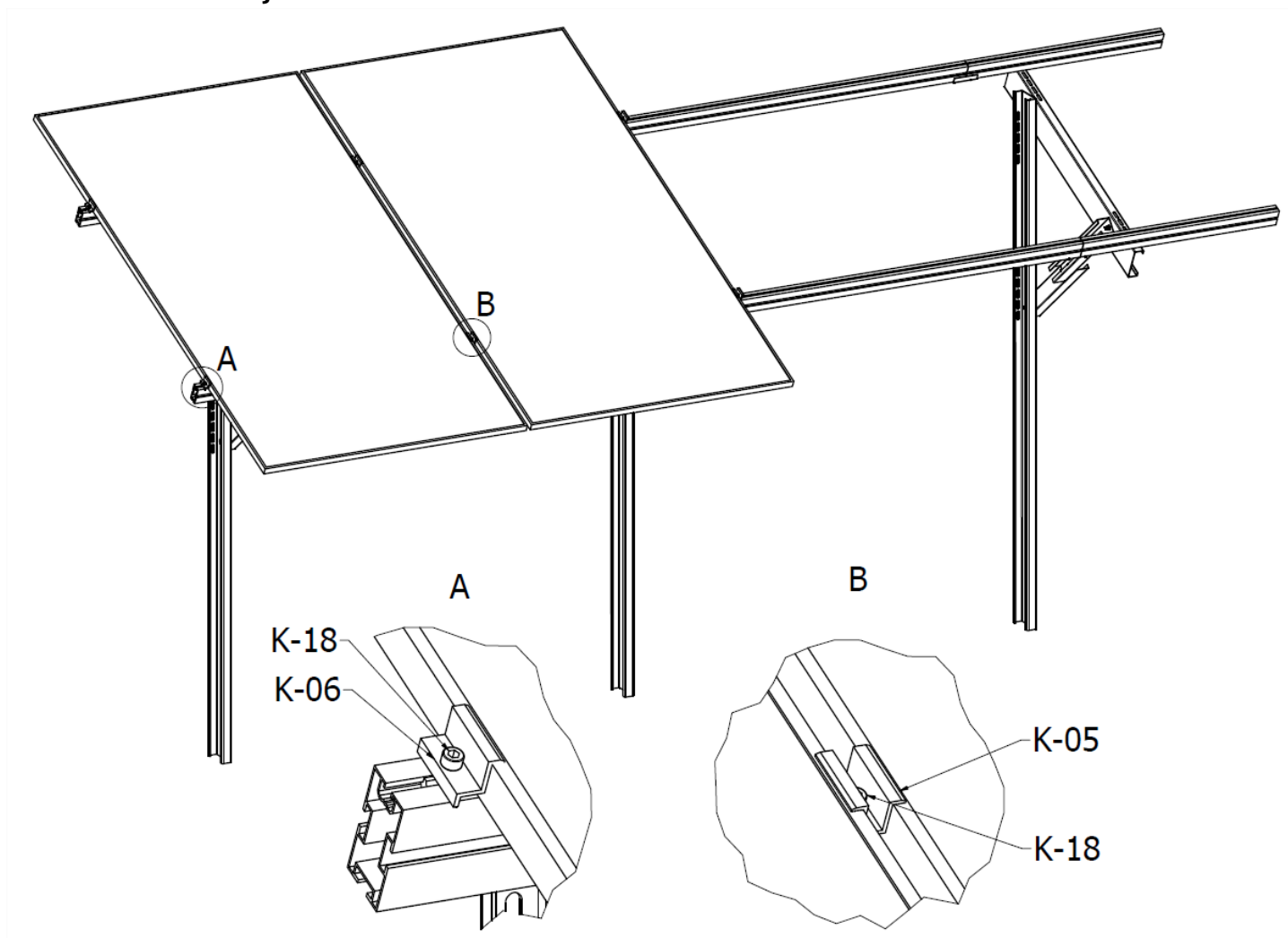
RYS.16. Montaż modułów i montaż klemy K-05 i K-06
