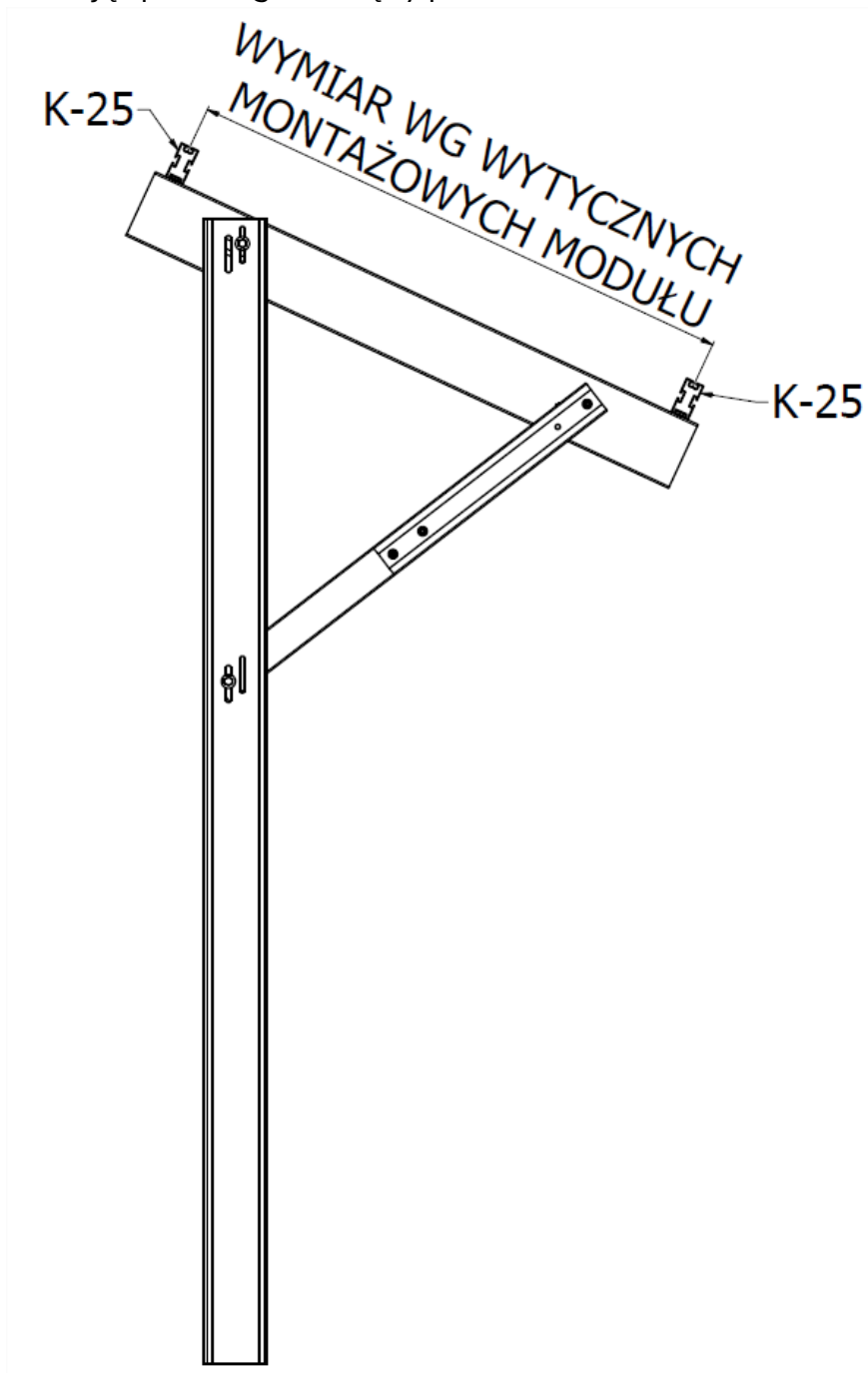
RYS.14. Rozstaw profili montażowych K-25
