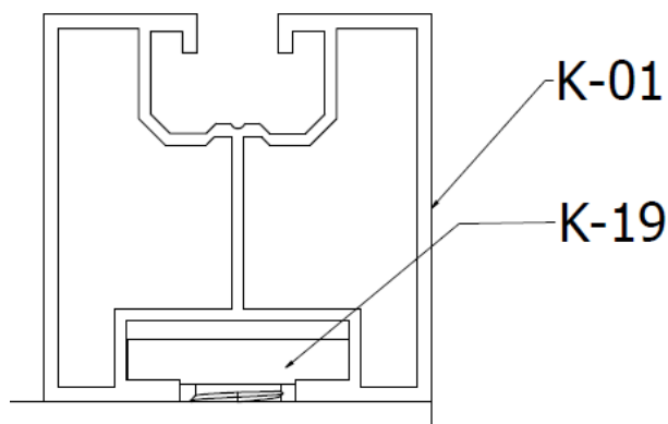
RYS.19. Montaż profilu K-01 (rzut II)
