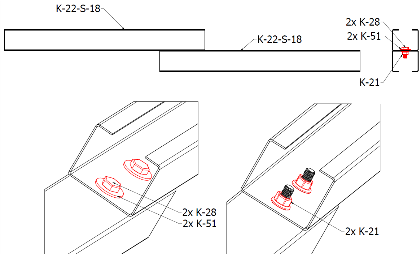
RYS.6. Skręcanie ramion
