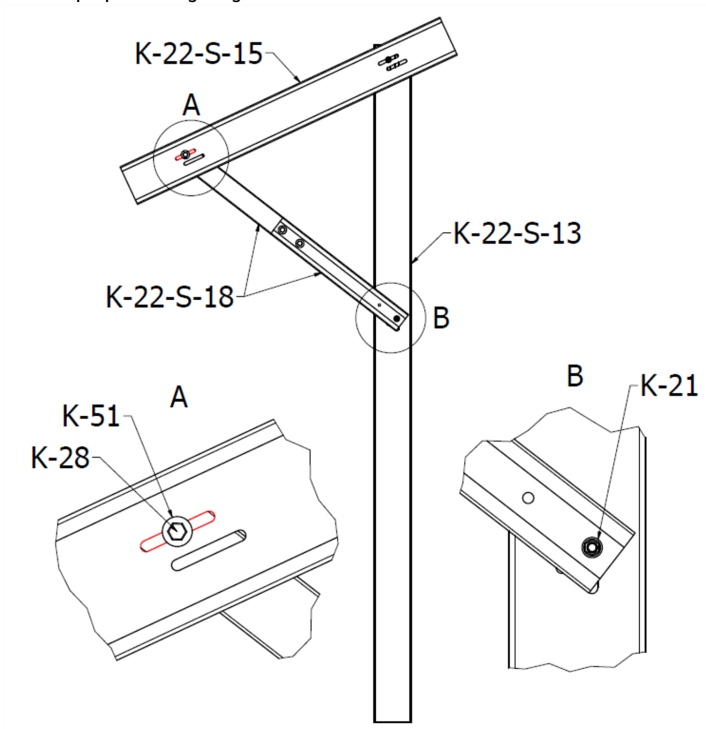
RYS.7. Montaż dłuższego ramienia do krokwi i podpory (rzut I)
