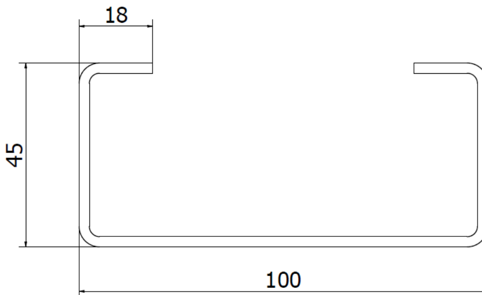
RYS.1. Przekrój podpory wbijanej w grunt
