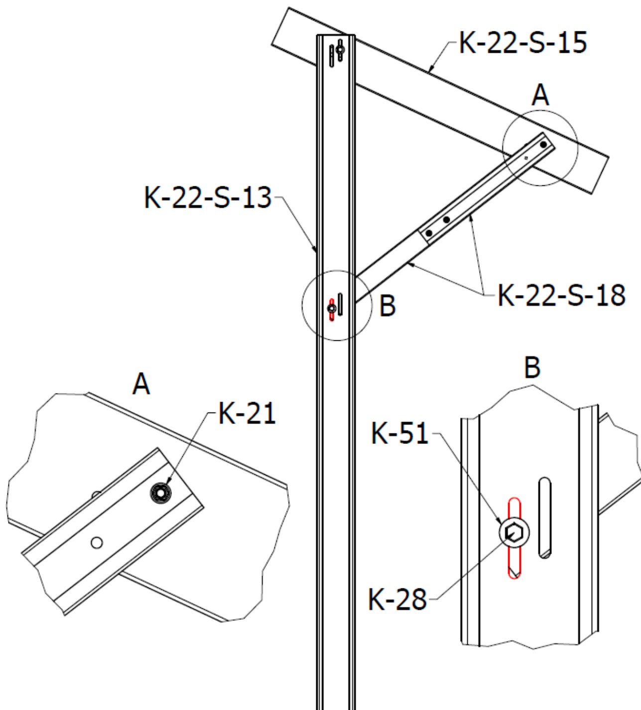
RYS.8. Montaż dłuższego ramienia do krokwi i podpory (rzut II)
