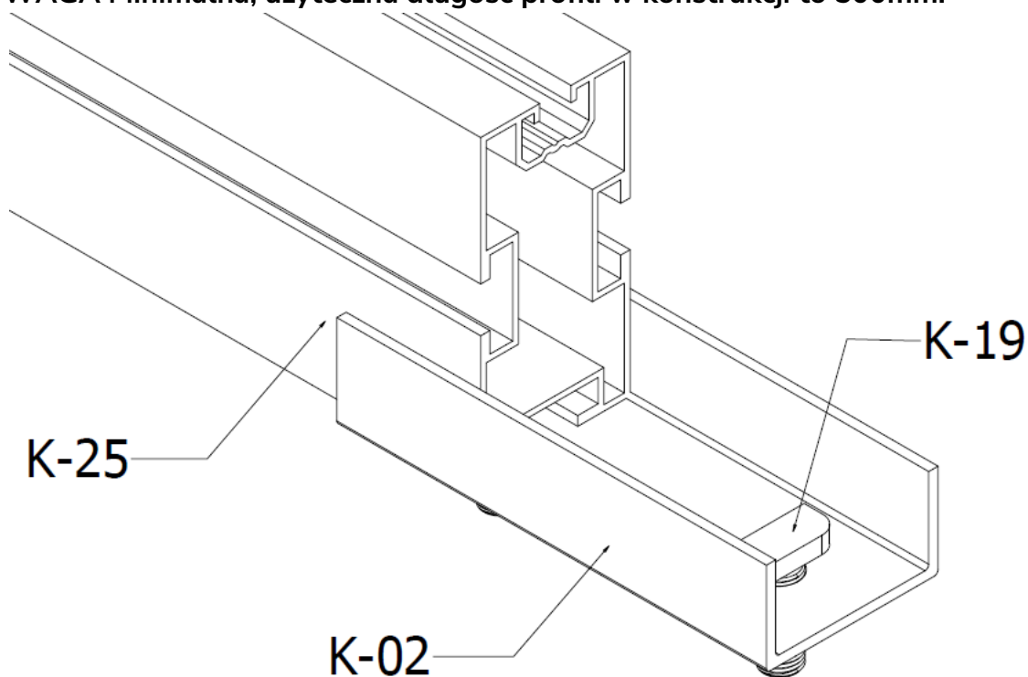
RYS. 9. Montaż łącznika K-02 z profilem K-25
