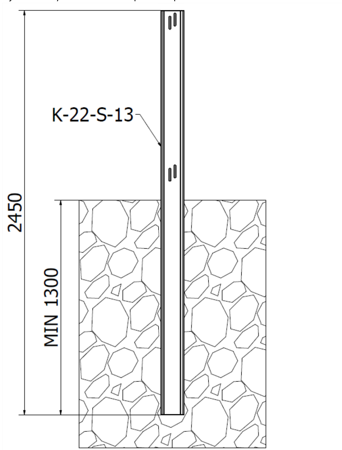
RYS.4. Montaż podpór w gruncie
