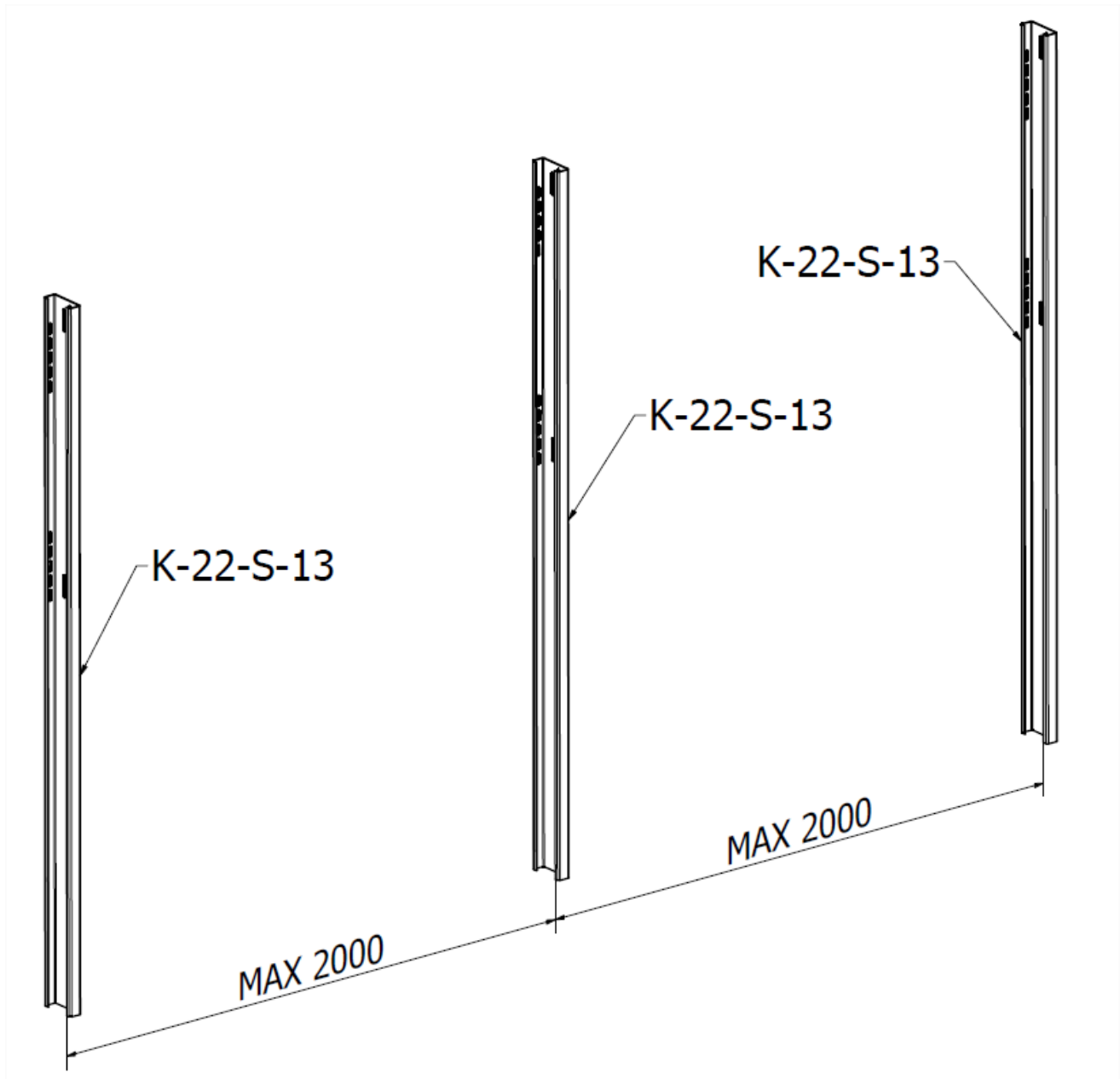
RYS.3. Rozstaw podpór
