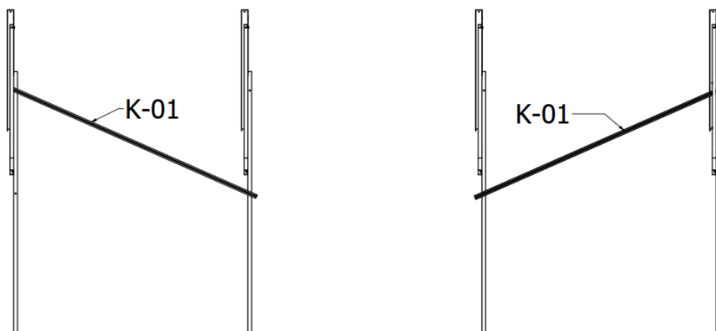
RYS.17. Widok zamontowanych zastrzałów do podpór K-22-S-13
