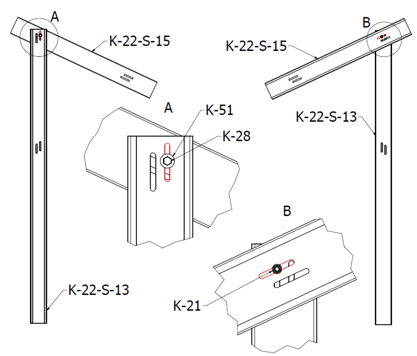
RYS..5. Montaż krokwi z podporą
