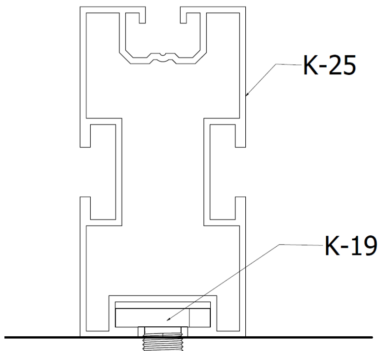
RYS.13. Montaż profilu K-25
