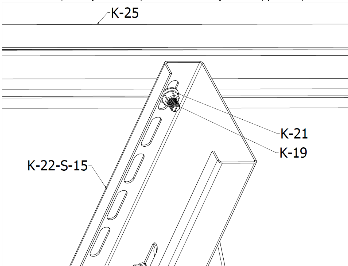
RYS.12. Montaż profilu K-25 do krokwi K-22-S-15
