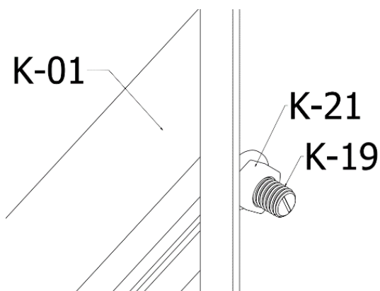
RYS.18. Montaż profilu K-01 (rzut I)
