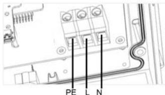
Ilustracja 13: Styki AC falownika jednofazowego
