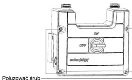
Ilustracja 38: Otwieranie pokrywę modułu zabezpieczającego DC:
