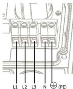
Ilustracja 14: Styki AC falownika trójfazowego
