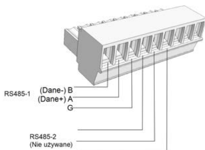
Ilustracja 25: Zacisk RS485
