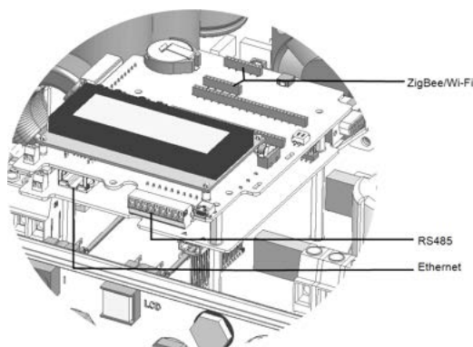
Ilustracja 19: Wewnętrzne złącza
