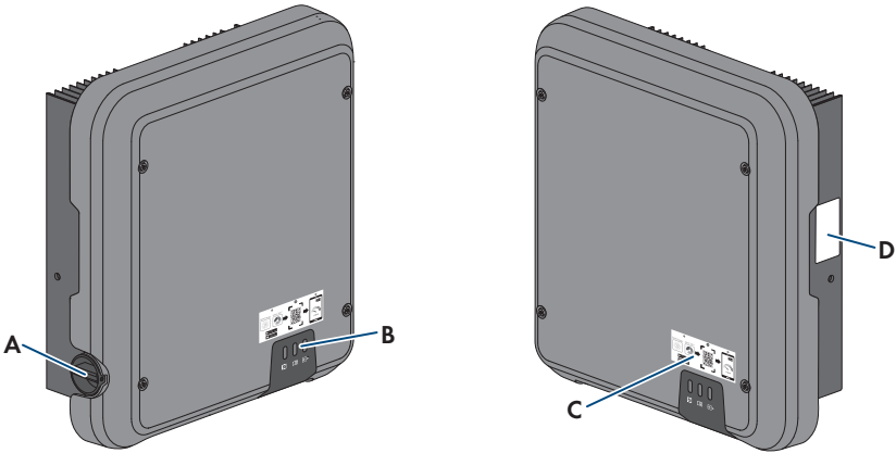
Ilustracja 2: Konstrukcja produktu
