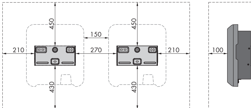
Ilustracja 8: Zalecane odstępy (wymiar w mm)
