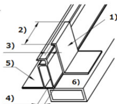
Rys. 4. Wymagania dotyczące klamer (zacisków)
