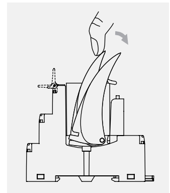
Sposób wyjmowania przekaźnika z gniazda przy pomocy obejmy wyrzutnikowej
