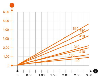
Wykres obciążenia wspornika typ AS 30
