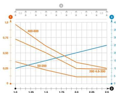
Diagram obciążenia korytka siatkowego GR-Magic typu GRM 55
