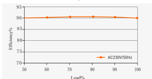
wydajność vs obciążenie / efficiency vs load
