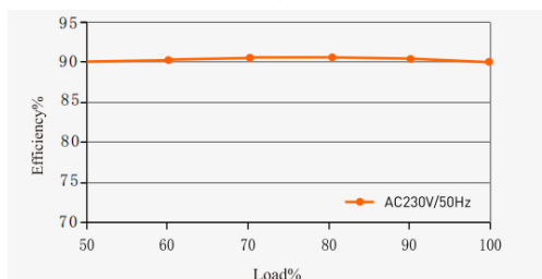
wydajność vs obciążenie / efficiency vs load
