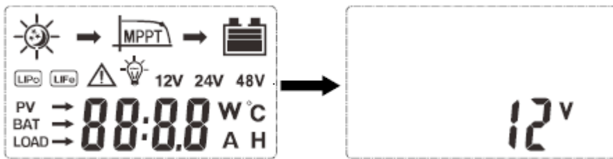
Interfejs początkowy
