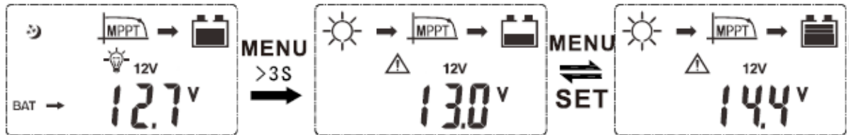
Strona główna
