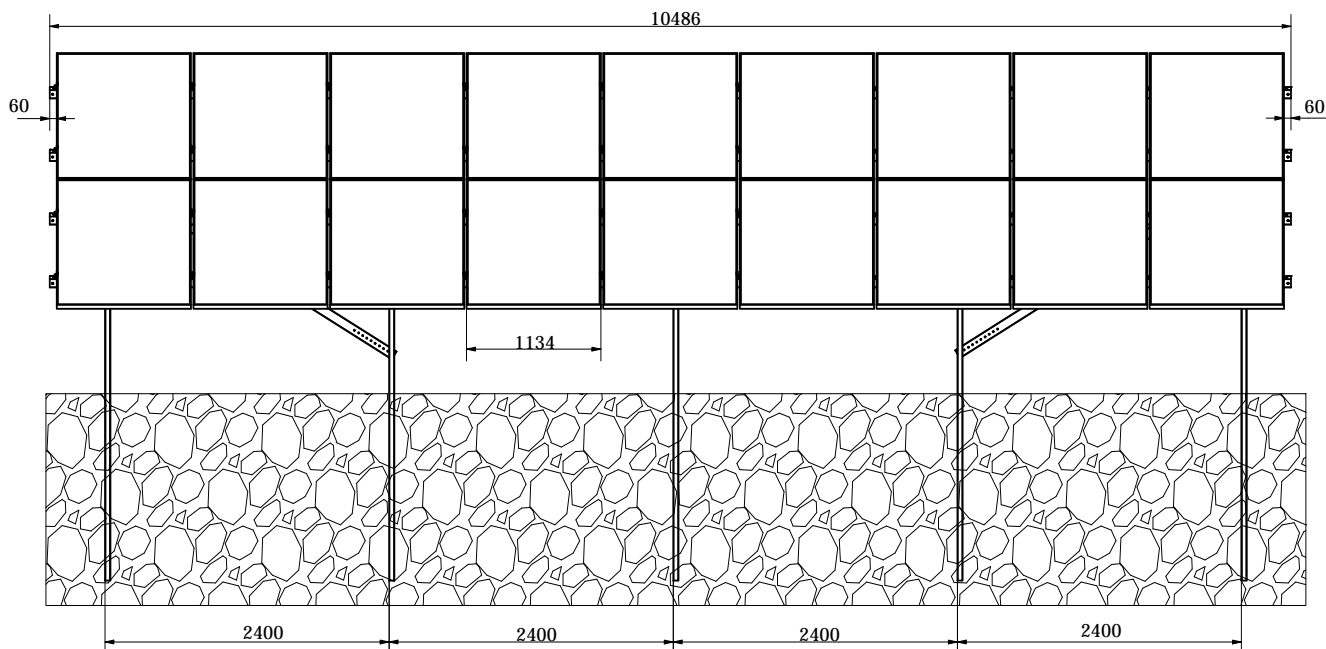
2 PION - 18 MODUŁÓW O SZEROKOŚCI 1134 [mm]
