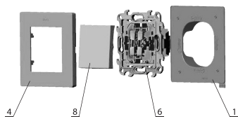
Łącznik pojedynczy/schodowy
