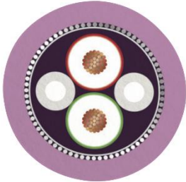
Kabelquerschnitt
