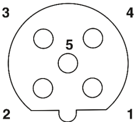
Polbild M12-Buchse, 5-polig, B-kodiert, Ansicht Buchsenseite
