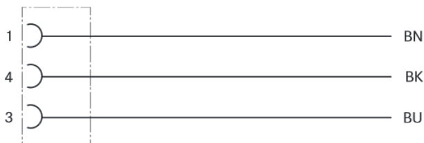
Schaltplan
