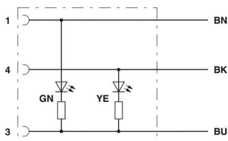
Kontaktbelegung der M12-Buchse mit LED
