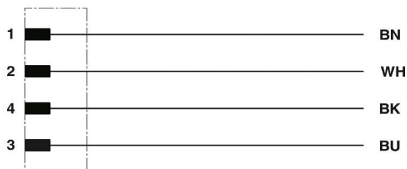
Schaltplan
