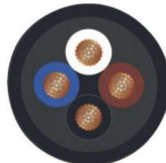
Kabelquerschnitt
