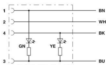
Kontaktbelegung der M12-Buchse mit LED
