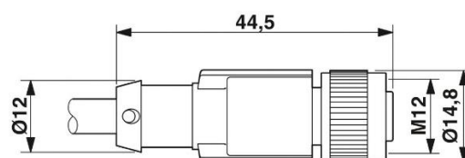
Buchse M12 x 1, gerade
