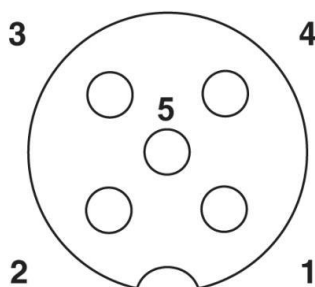
Polbild M12-Buchse, 5-polig, A-kodiert, Ansicht Buchsenseite
