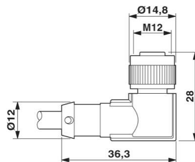
Buchse M12 x 1, gewinkelt
