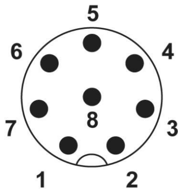
Polbild M12-Stecker, 8-polig, Ansicht Stiftseite
