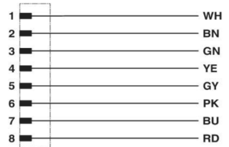
Kontaktbelegung des M12-Steckers
