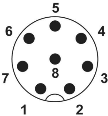
Polbild M12-Stecker, 8-polig, Ansicht Stiftseite
