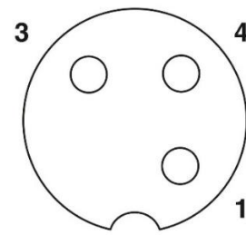
Polbild M12-Buchse, 3-polig, A-kodiert, Ansicht Buchsenseite
