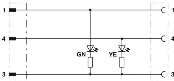
Kontaktbelegung des M12-Stecker und der M12-Buchse
