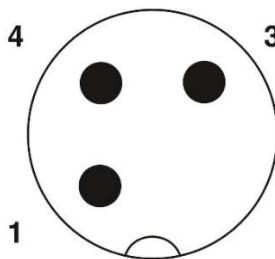
Polbild M12-Stecker, 3-polig, A-kodiert, Ansicht Stiftseite
