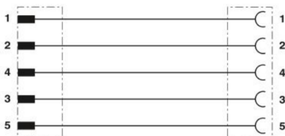
Schaltplan
