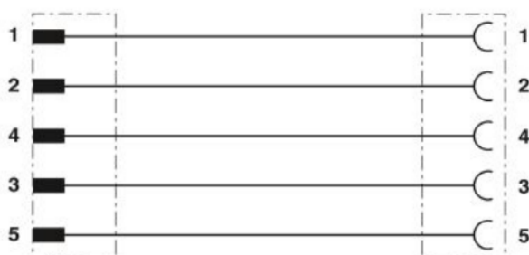
Schaltplan
