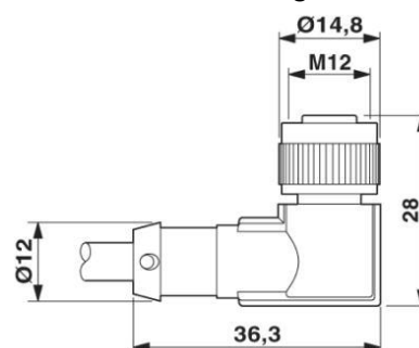
Buchse M12 x 1, gewinkelt
