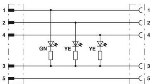
Schaltplan
