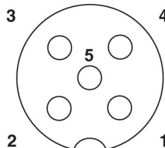
Schemazeichnung
