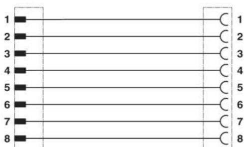
Kontaktbelegung des M12-Stecker und der M12-Buchse
