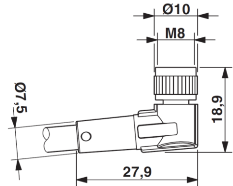
Buchse M8 x 1, gewinkelt
