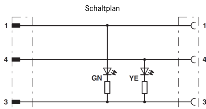
Kontaktbelegung der M12-Stecker/M8-Buchse
