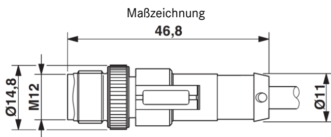
M12-Stecker, 3-polig, A-kodiert
