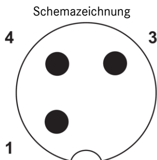
M12-Stecker, 3-polig, A-kodiert
