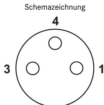
Buchse M8, 3-polig, A-kodiert
