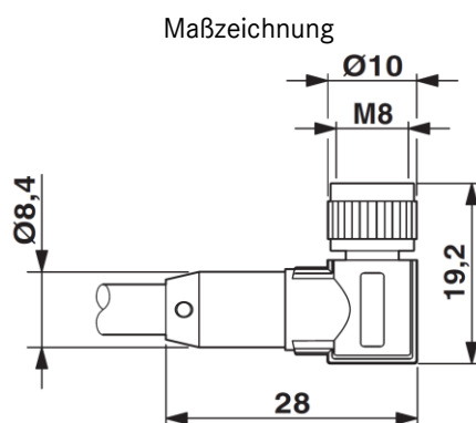
Buchse M8 x 1, gewinkelt, mit LED
